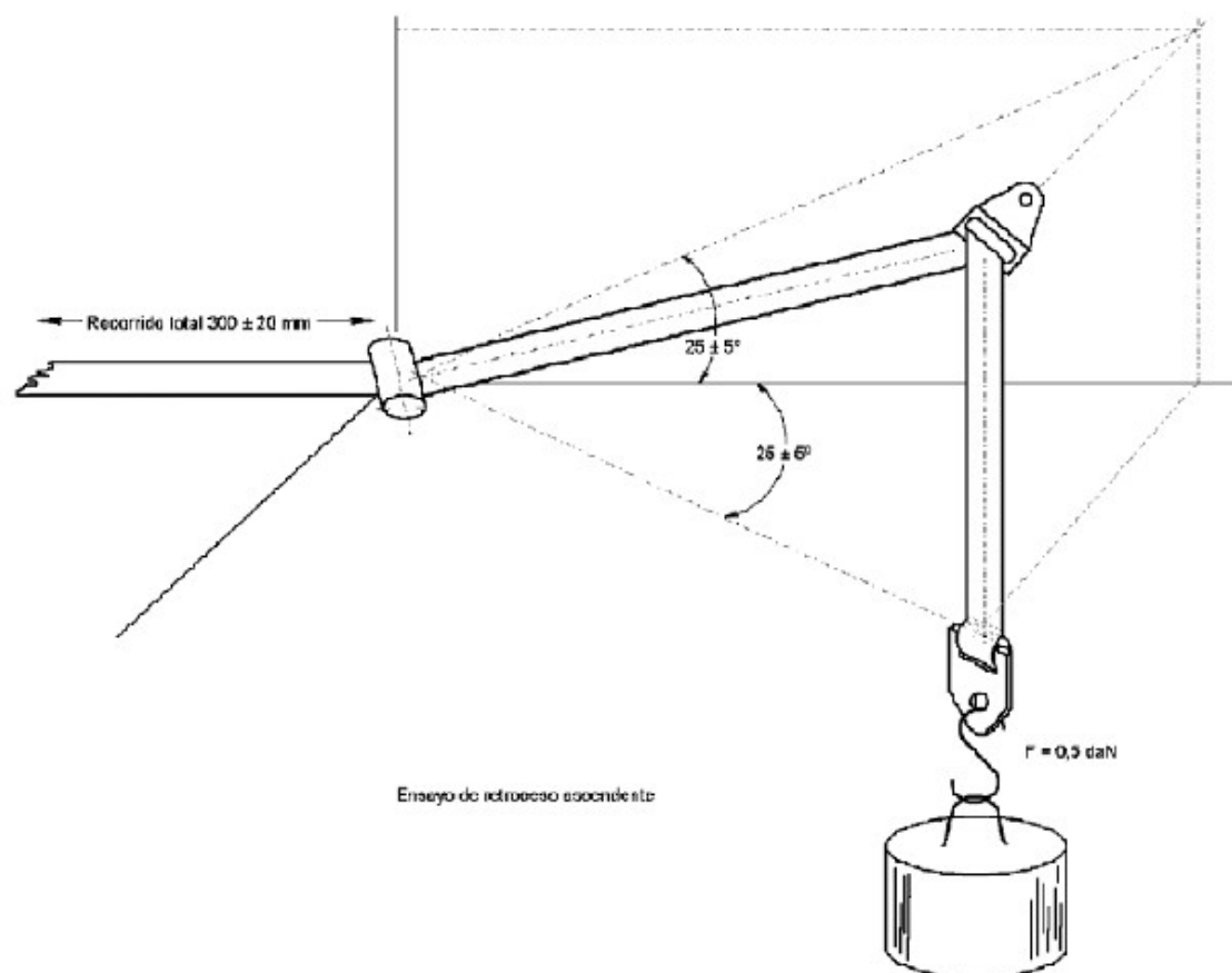
Figura 3- Procedimiento Clase 3 y prueba de micro-deslizamiento
