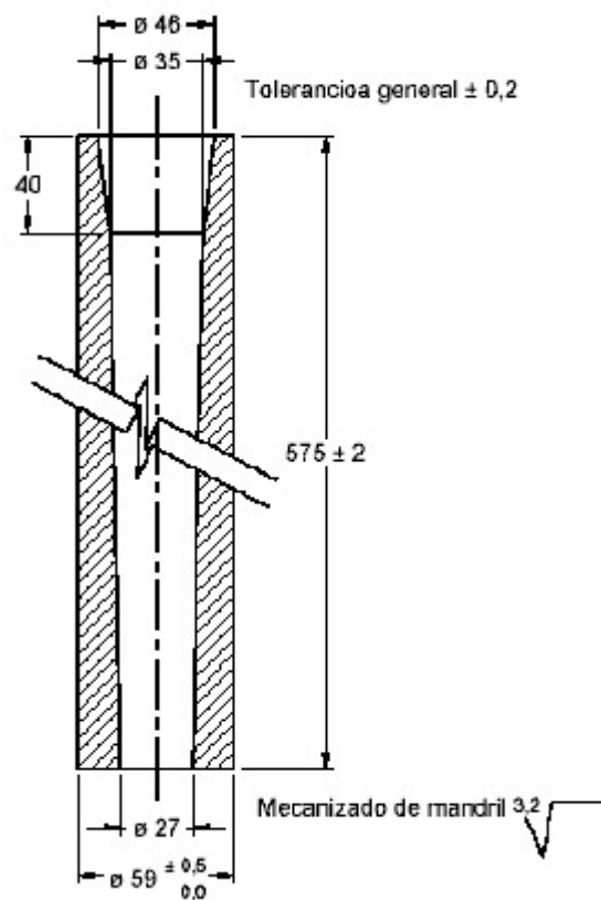
Figura 3. Dispositivo de freno (tubo de poliuretano)
