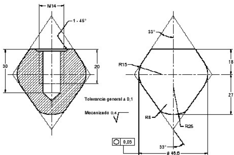
Figura 4. Dispositivo de freno (mango ovalado)
