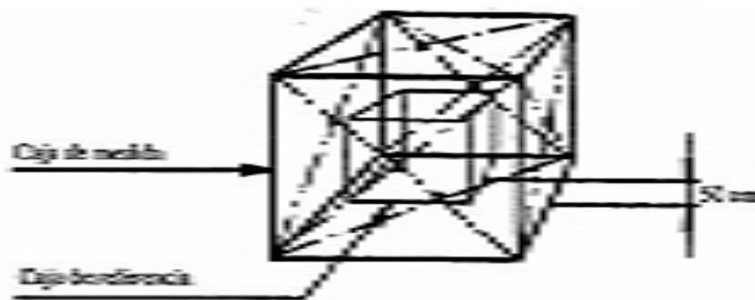
Figura F.2. Emplazamientos de micrófono para juguetes de mano, distintos a los juguetes con fulminantes.
