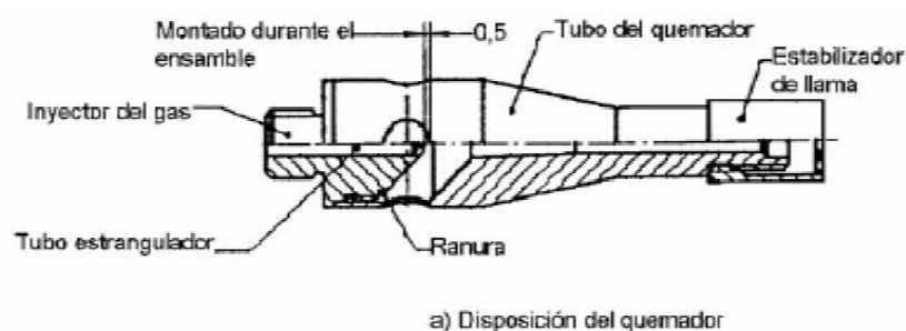
Figura 1 Quemador
