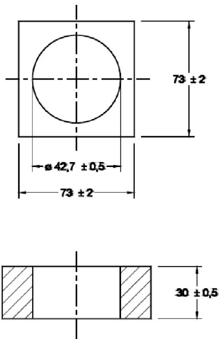
Figura 15. Plantilla complementaria de ensayo B 5.4 Ensayo para pelotas pequeñas (véase numeral 4.5.2)
