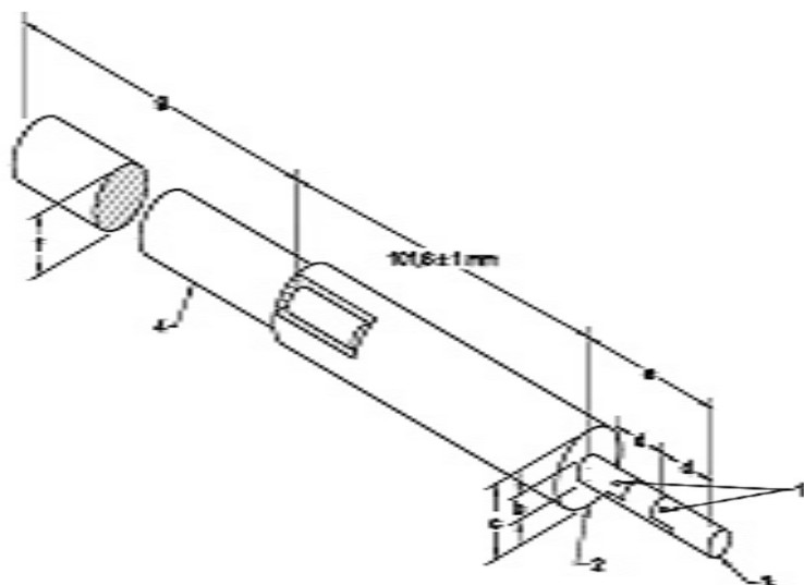
Figura 17. Sonda de accesibilidad.
